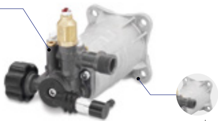
accoppiamento diretto pompa/motore a scoppio direct coupling pump with gasoline motor drive
